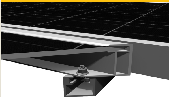
Beispiel 2 - Verschraubung direkt
